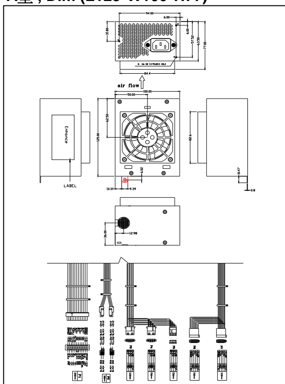
A型 , Dim (L125*W100*H77)
