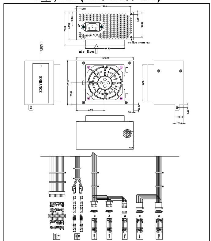
D型 , Dim (L125*W100*H77)
