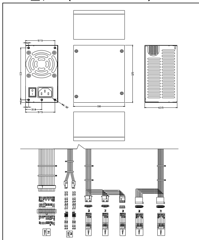
F型 , Dim (L125*W100*H63.5)
