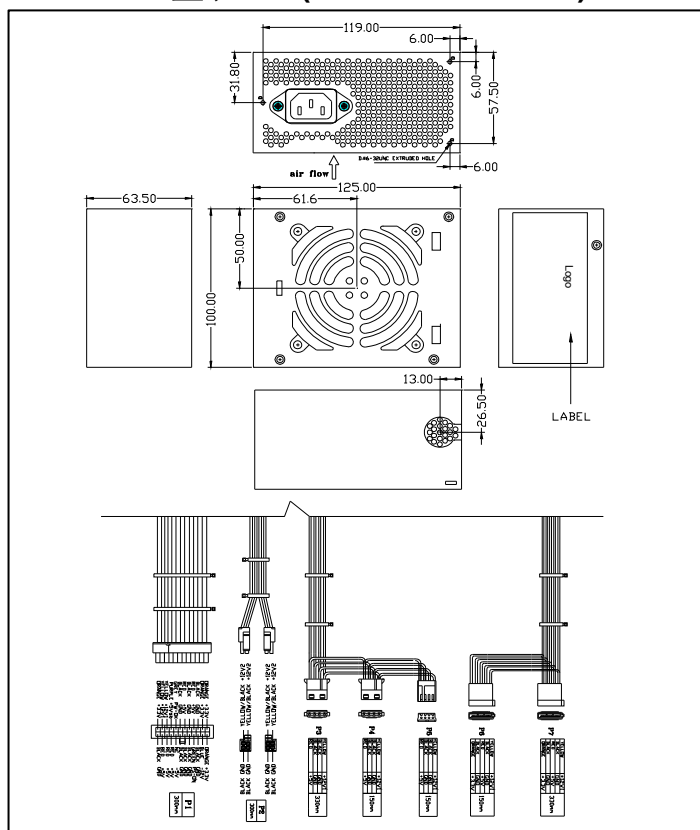
H型 , Dim (L125*W100*H63.5)
